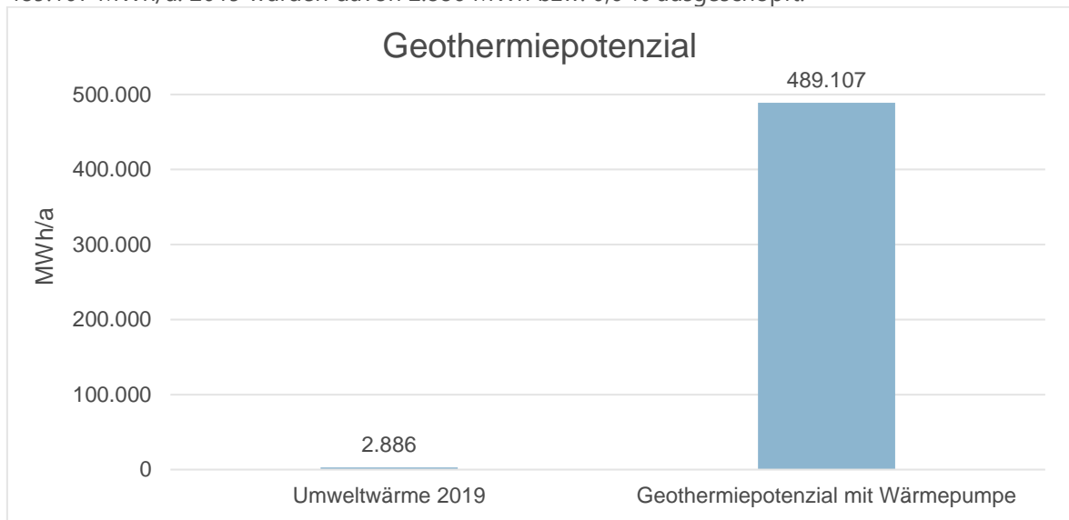
Abbildung 39: Geothermiepotenzial Aurich
